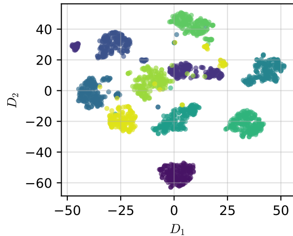
t-SNE, perplexité = 30
