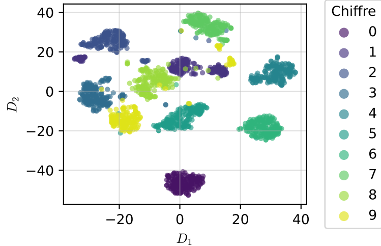
t-SNE, perplexité = 50
