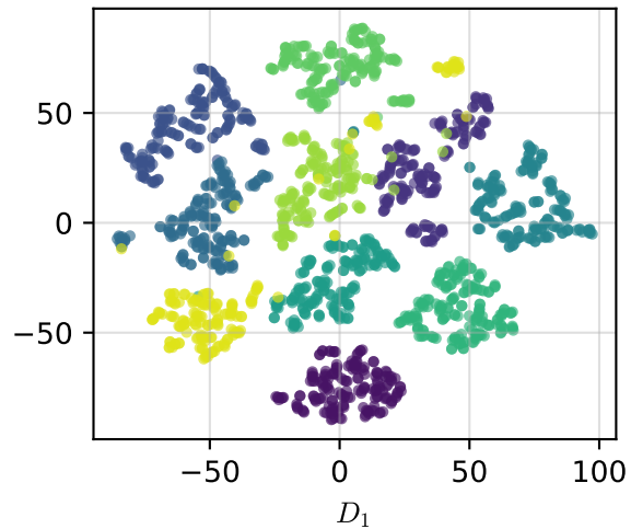
t-SNE, perplexité = 5
